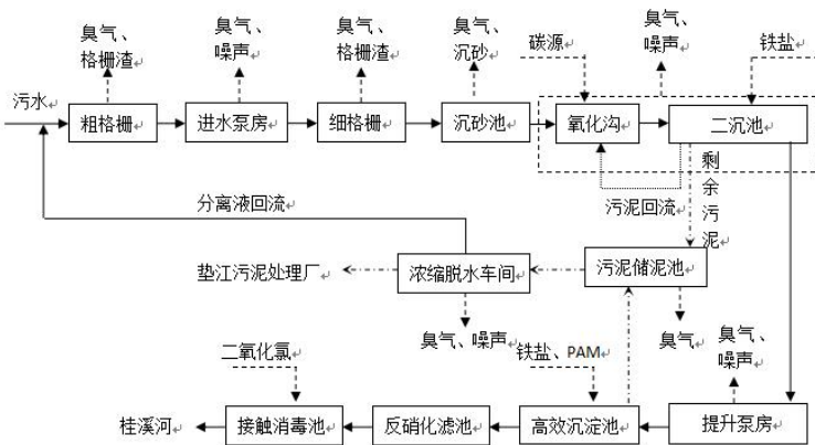
图 2.13-1 污水处理厂工艺流程图
