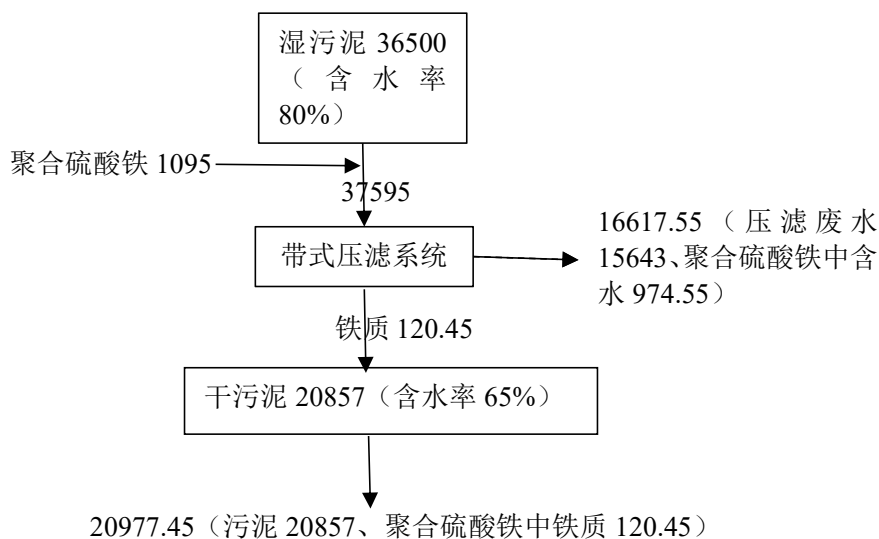
2.8-1 项目建成后全厂物料平衡图（单位：t/a）
