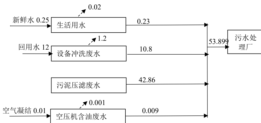
图 2.7-1 项目水平衡图 单位：m³/d
