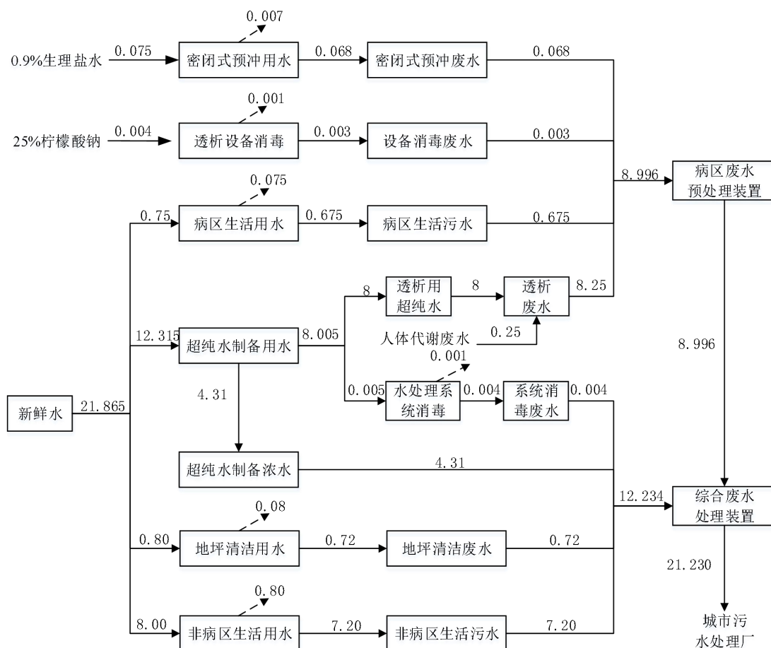
图 2.1-1 项目用排水量平衡图 单位：m³/d
