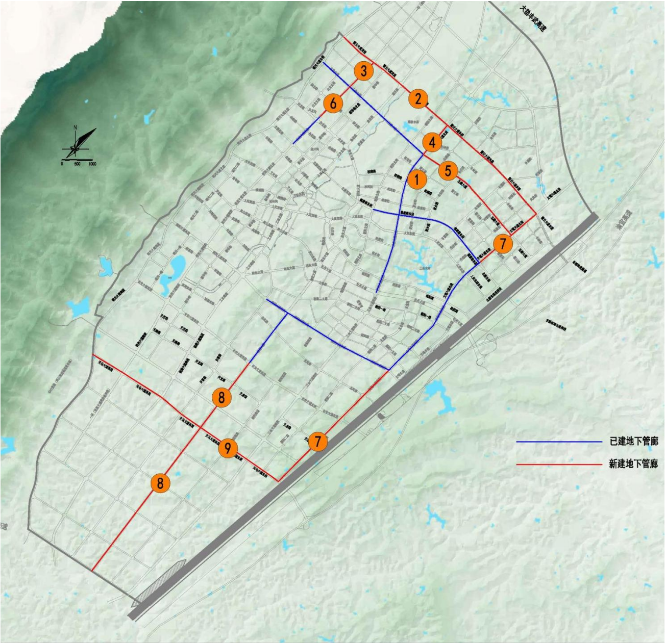
综合管廊规划图 综合管廊项目规划表
