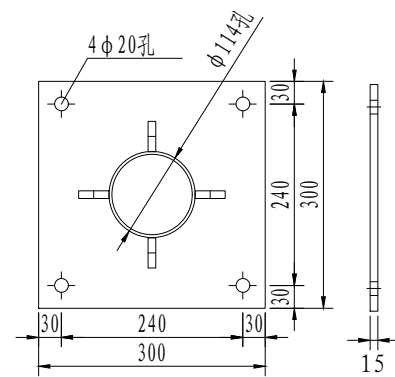
加劲法兰盘
