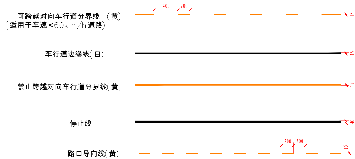
标线线形
