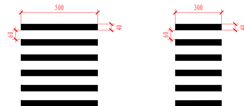
人行横道线
