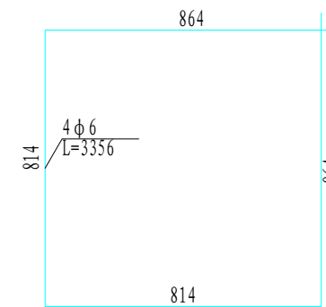
箍筋大样图
