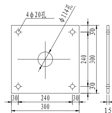
底座法兰盘
