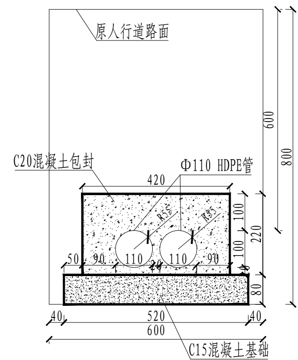
人行道开挖穿线管暗敷管道剖面图 (沿人行道每3米包封一处, 每处包封长0.3米)
