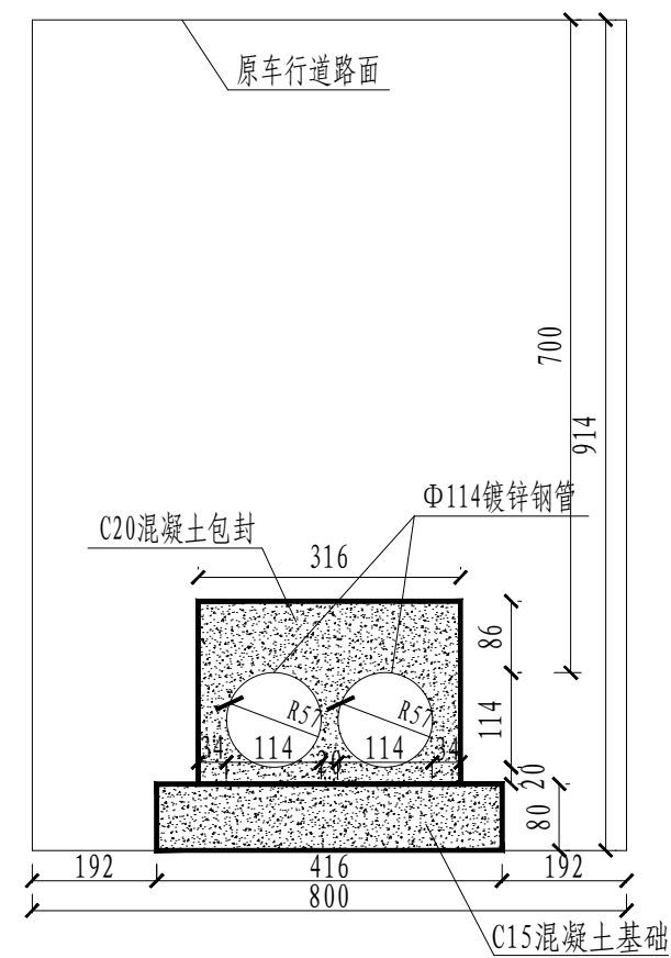
机动车道开挖穿线管暗敷管道剖面图 (沿车行道通长包封)
