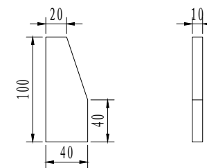
底座加劲肋
