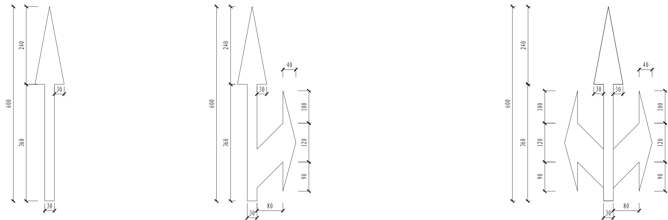
6m 导向箭头大样图
