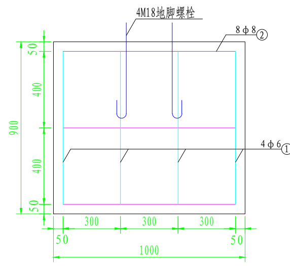
基础配筋图
