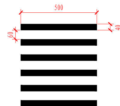
人行横道线
