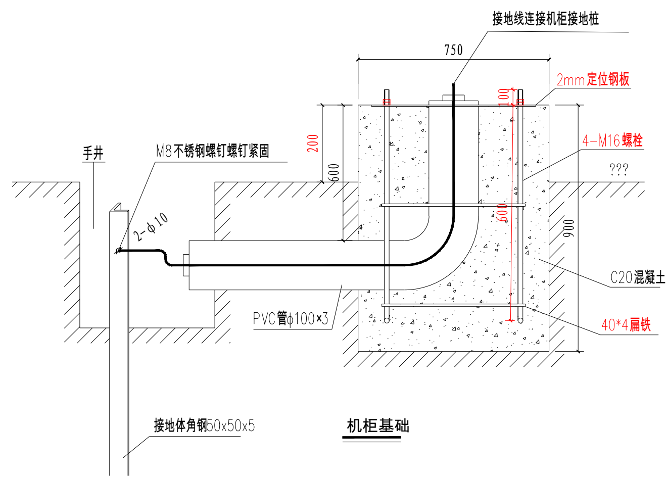
正视图
