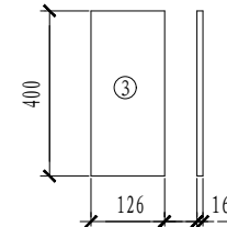
节点板大样图
