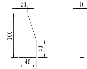
底座加劲肋
