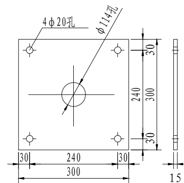
底座法兰盘
