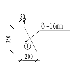
立柱加筋肋大样图
