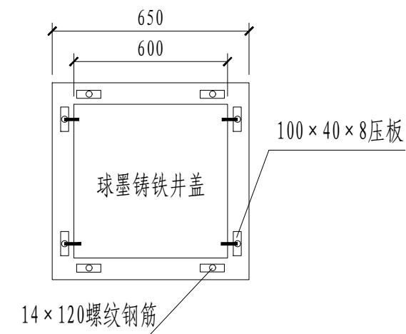
井盖平面图
