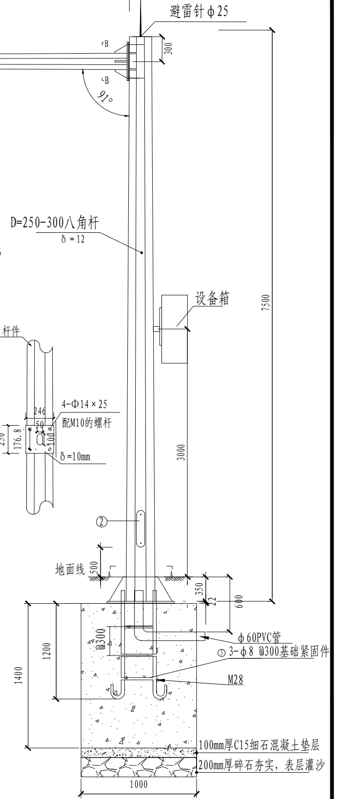
电子警察杆件大样图
