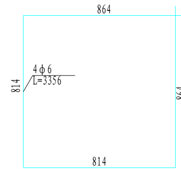
箍筋大样图
