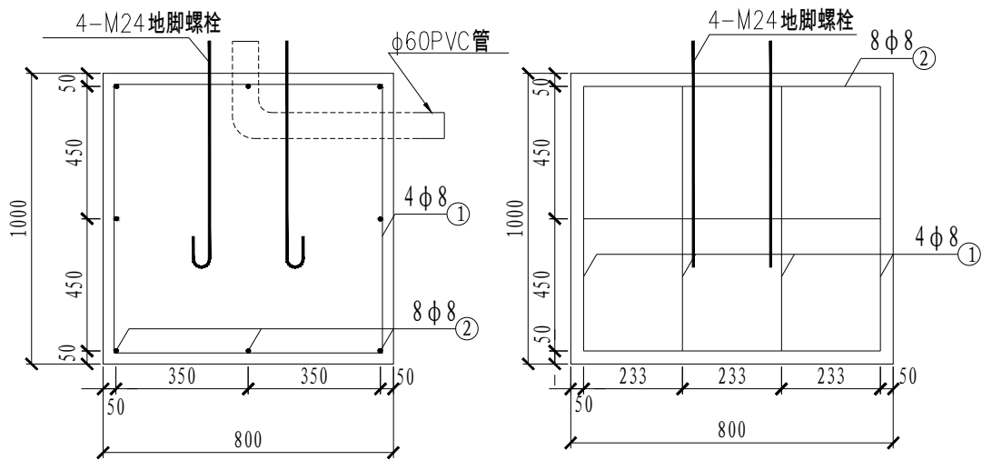
基础配筋图
