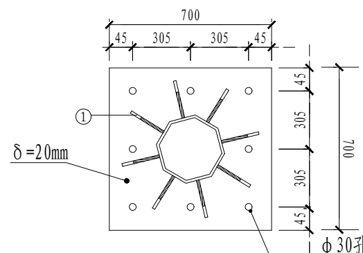
底座法兰盘
