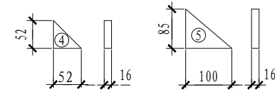
横梁加筋肋大样图
