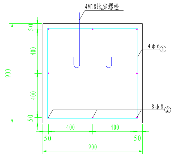
基础配筋图
