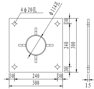
加劲法兰盘
