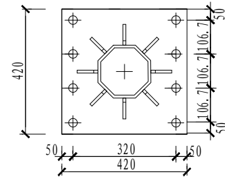
B-B断面
