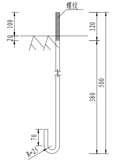
地脚大样图
