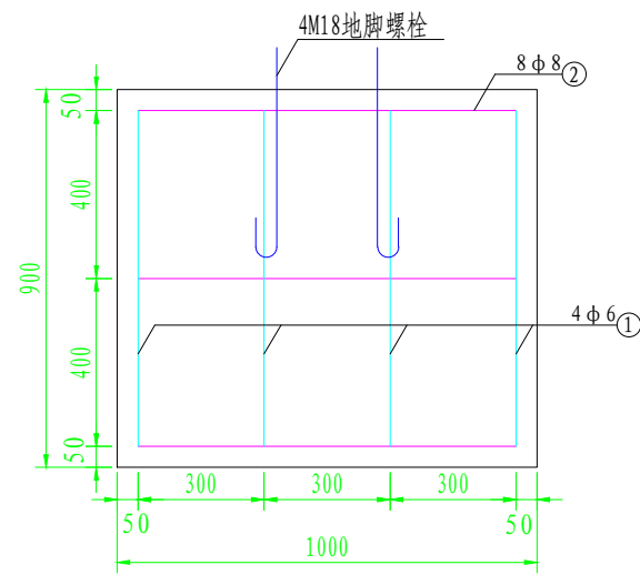
基础配筋图
