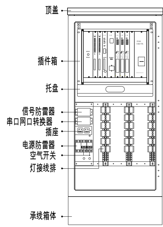
内部布置图
