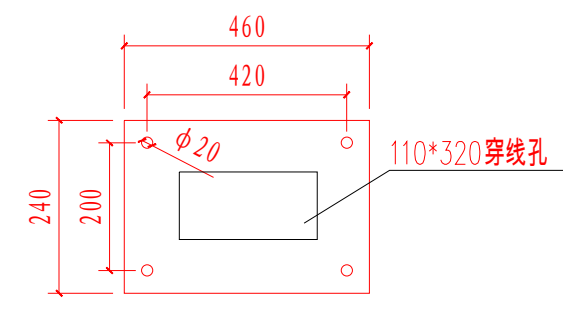
定位钢板平面
