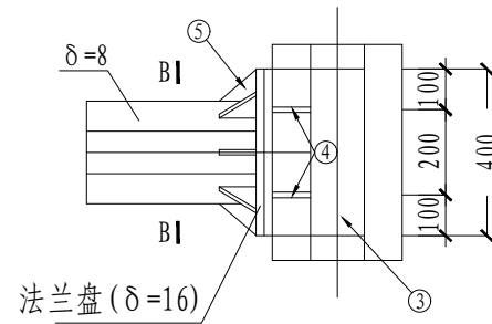
横梁与端梁连接详图
