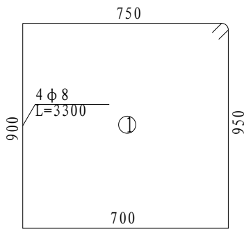
① 箍筋大样图
