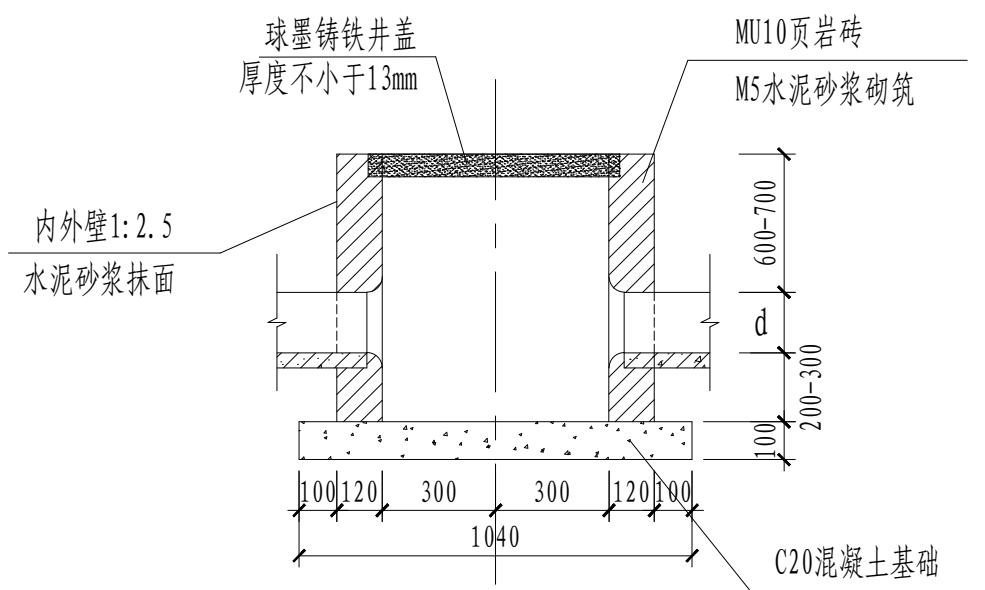
沙井剖面图
